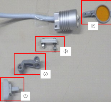
取付具組付状態
